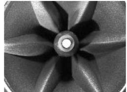
Abb.11: DBGM-geschützte Anordnung von LED- Scheuchblitzstrahler (-..X) im Zentrum des Scheuch-Strahlers.
